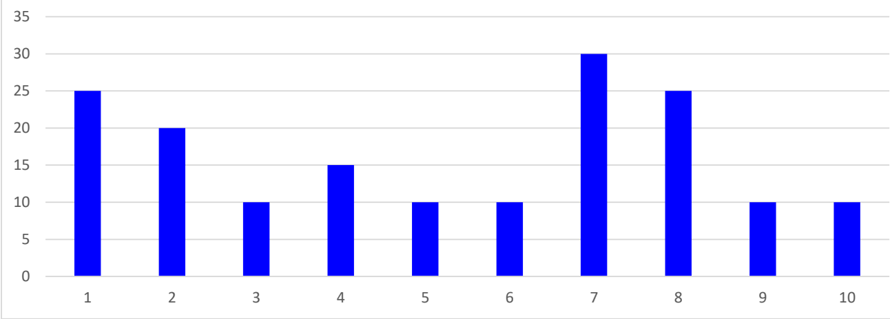
Pronóstico Acumulados de lluvias
