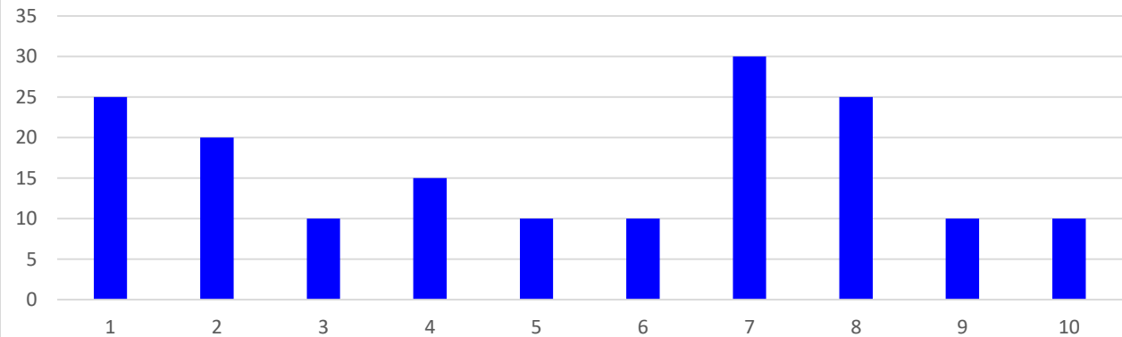
Pronóstico Acumulados de lluvias
